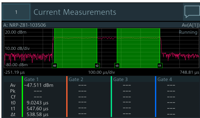
Определение мощности пакетного сигнала EDGE с помощью трехканального дидного датчика мощности R&S®NRPxxS(N) и функции стробирования; исключение тренировочной последовательности в центре сигнала
