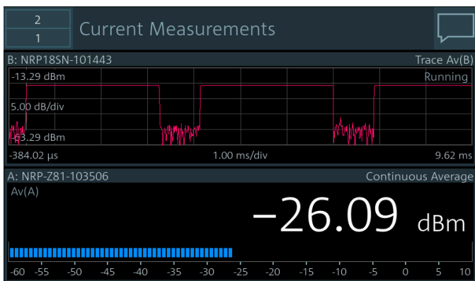
Совместное отображение измерительной кривой и результата непрерывного усреднения
