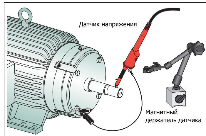
Рисунок 5. Настройка проверки вала двигателя
