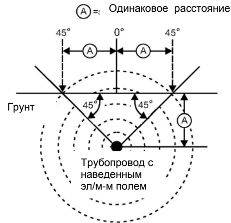
Рис. 8. Проверка искажения.
