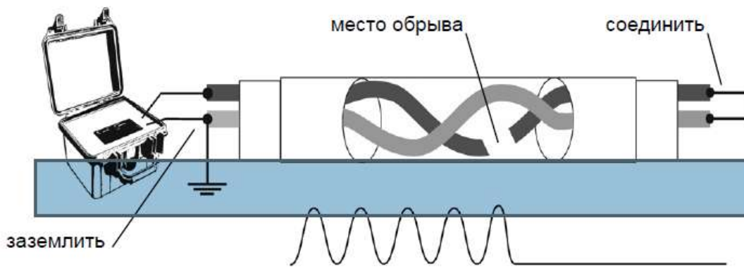
Рисунок 5.3.4.2 – Схема подключения и уровень сигнала при поиске обрыва в кабеле без экрана и брони
