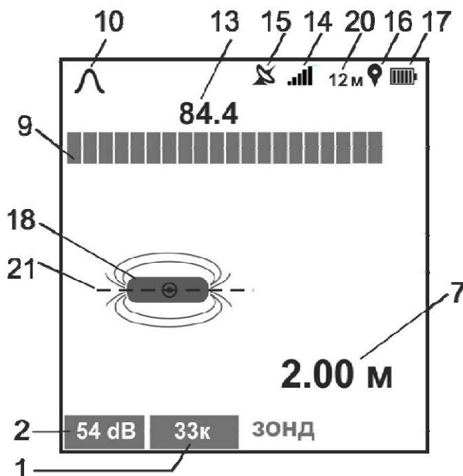
Рисунок 3.4 – Индикация приемника в режиме «ЗОНД»
