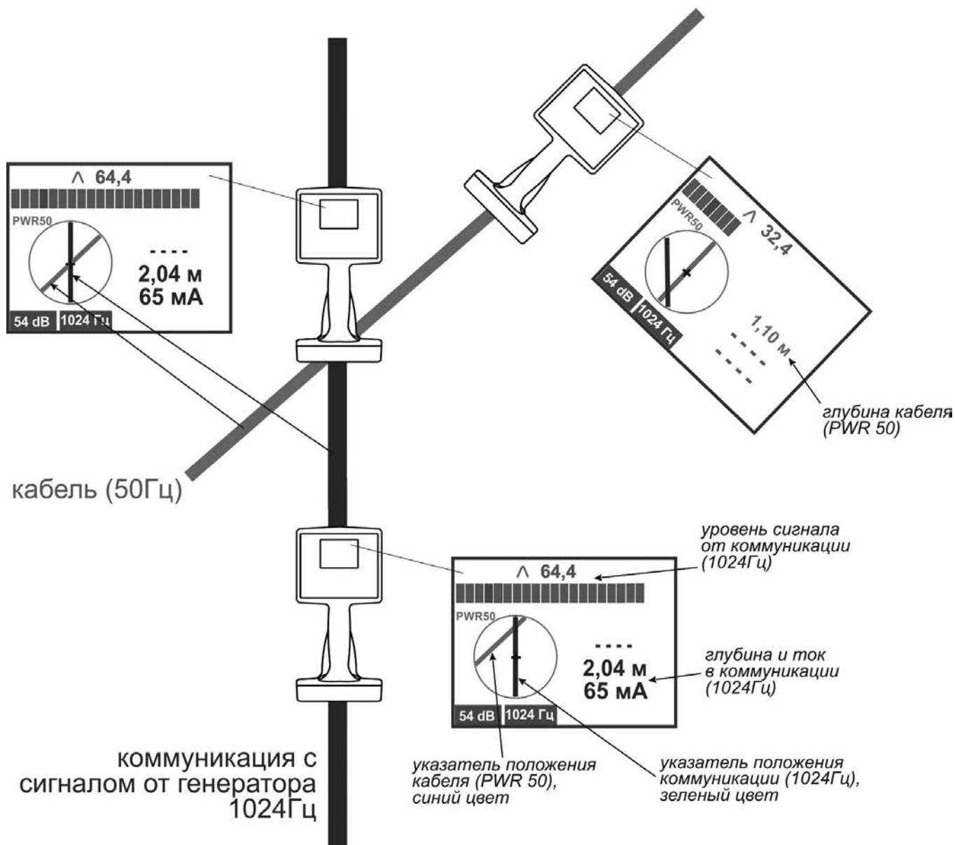
Рисунок 4.2.3 б – Поиск с включенной функцией «Вторая линия»
