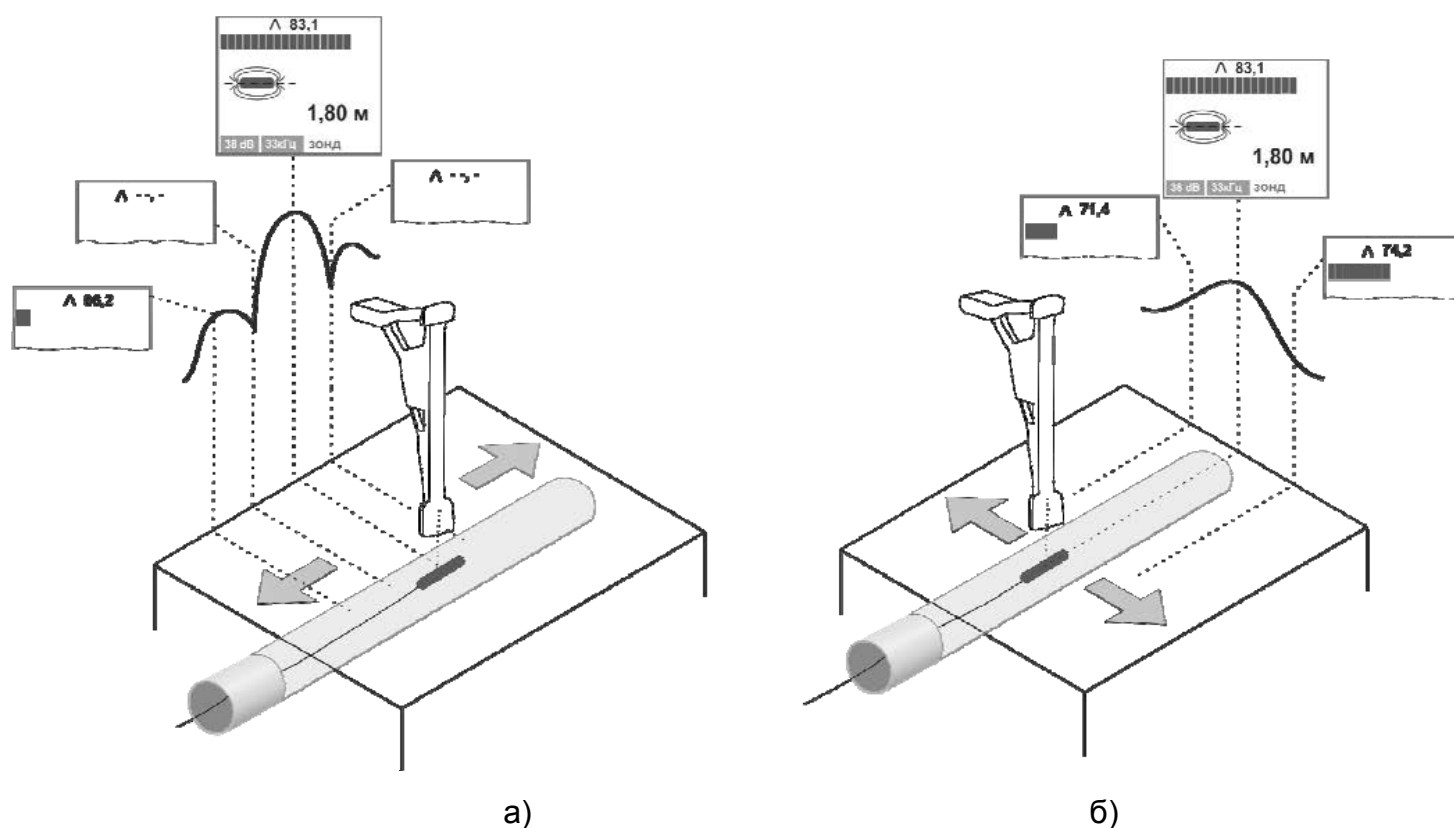
Рисунок 4.5.2 – Определение точного положения и глубины залегания зонда
