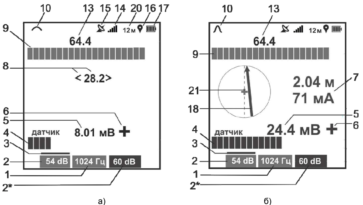
Рисунок 3.3 – Индикация приемника в режиме «ТРАССА-ДАТЧИК»
