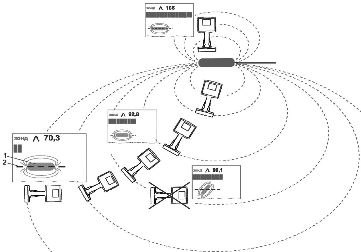
Рисунок 4.5.1 – Поиск местоположения зонда
