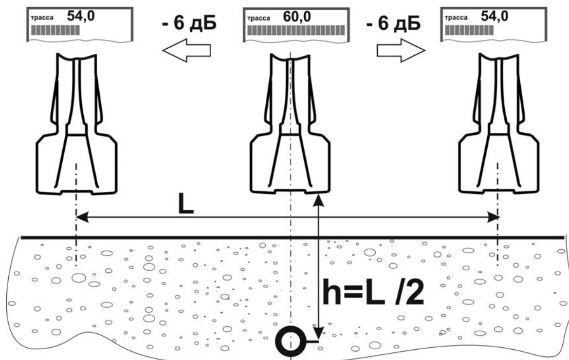
Рисунок 4.3.1 – Определение глубины залегания методом «-6дБ»
