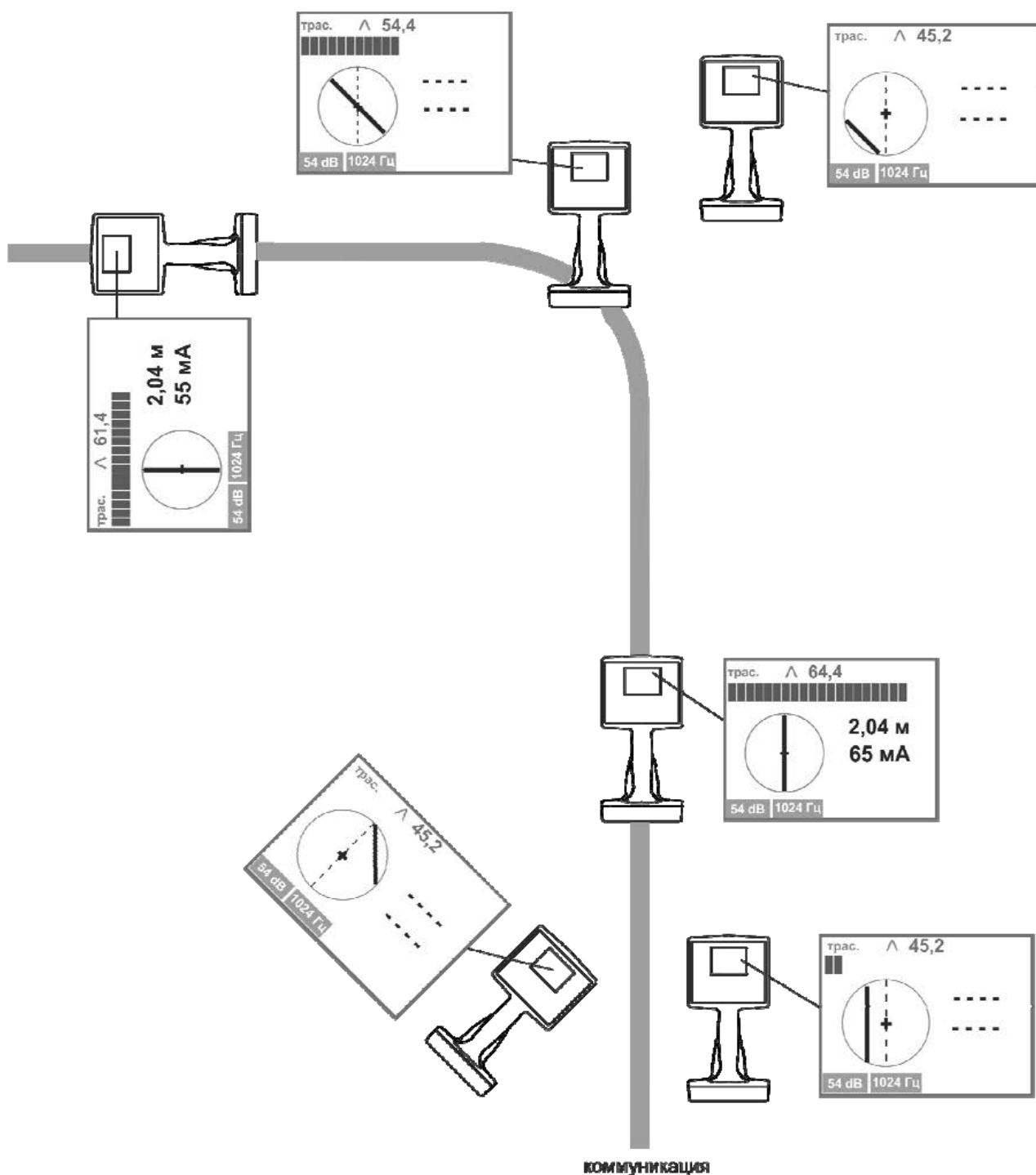
Рисунок 4.2.3 а – Поиск с включенной функцией «КОМПАС»
