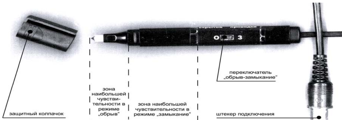
Рисунок 5.3.4.1 – Мини-датчик МД-01
