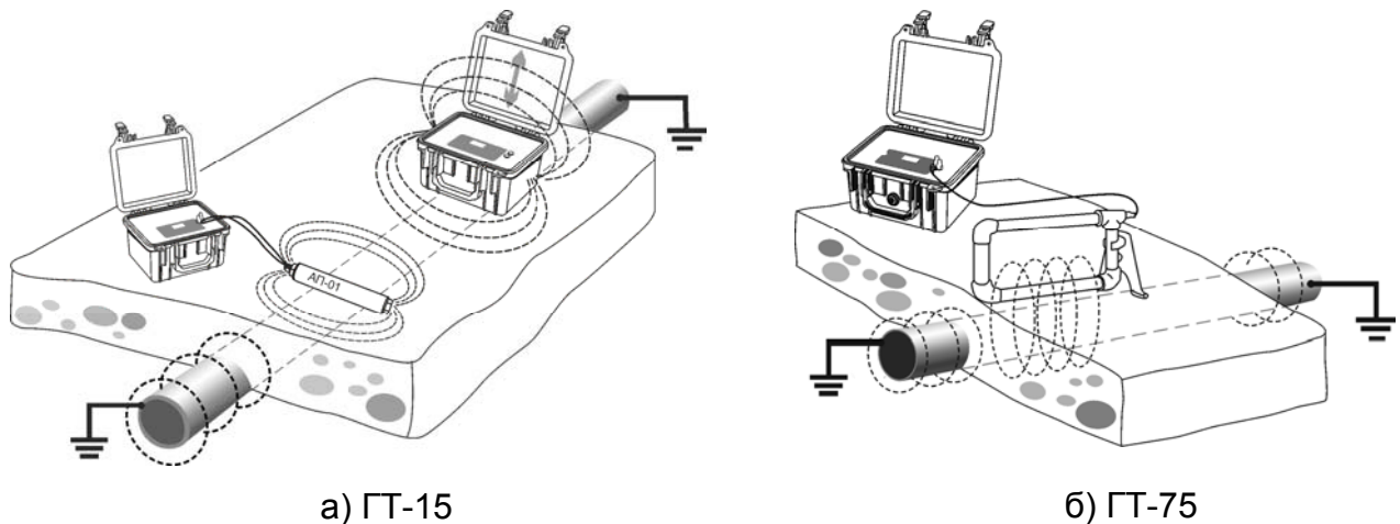
Рисунок 2.3.2 – Способы бесконтактного задания тока в коммуникации
